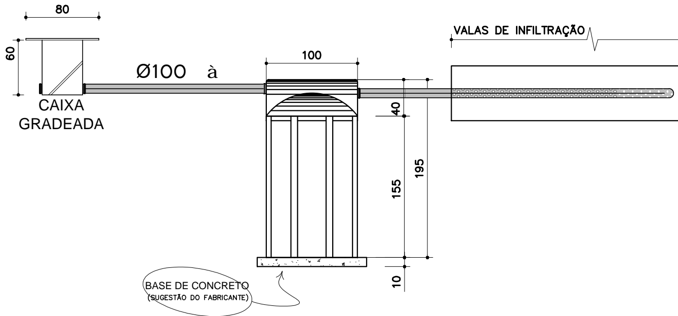
VISTA LATERAL
