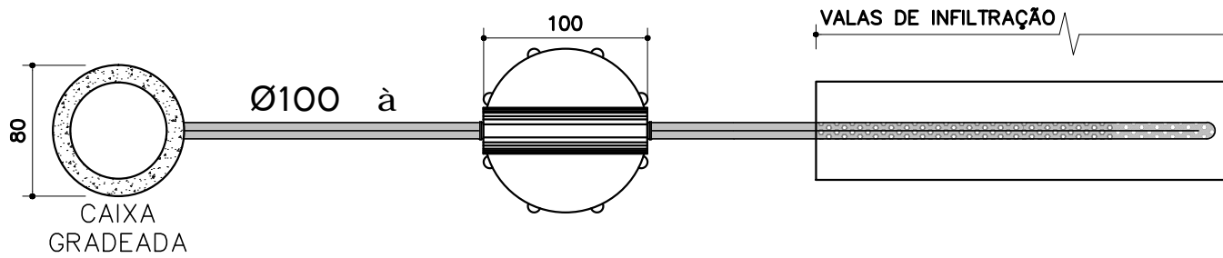
VISTA SUPERIOR
